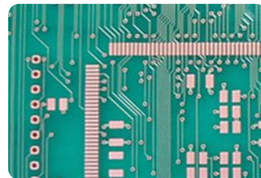
Solder Resist의 PATTERNING 후의 기판표면
