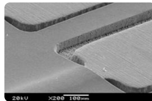
전자현미경 사진: 좌측이단이Solder Resist
