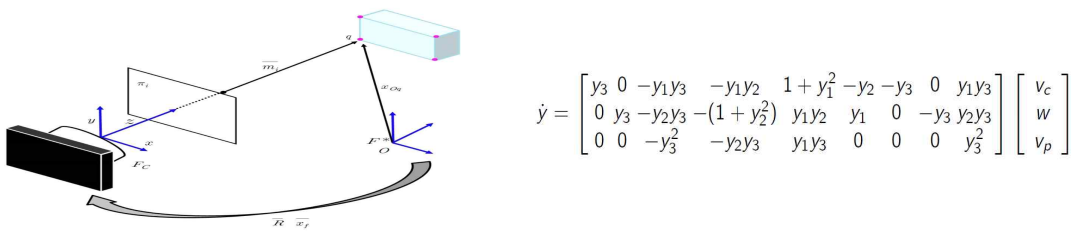
그림 3. 카메라와 목표물 사이의 좌표계.
